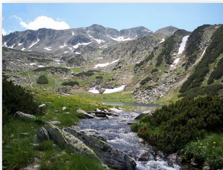
Creasta Retezatului
